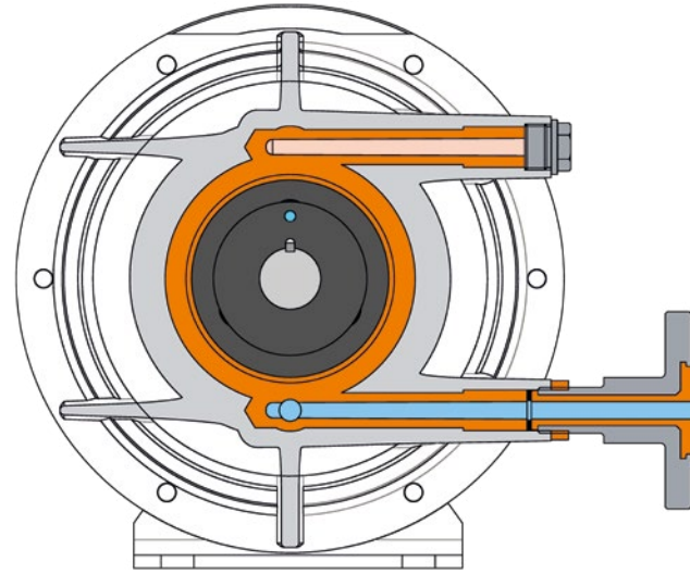
Spülanschluss für externe Gleitlagerschmierung
