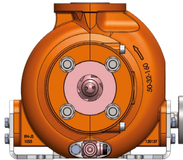
CM mit Spülanschluss und Ventil für Spiralgehäuse-Entleerung
